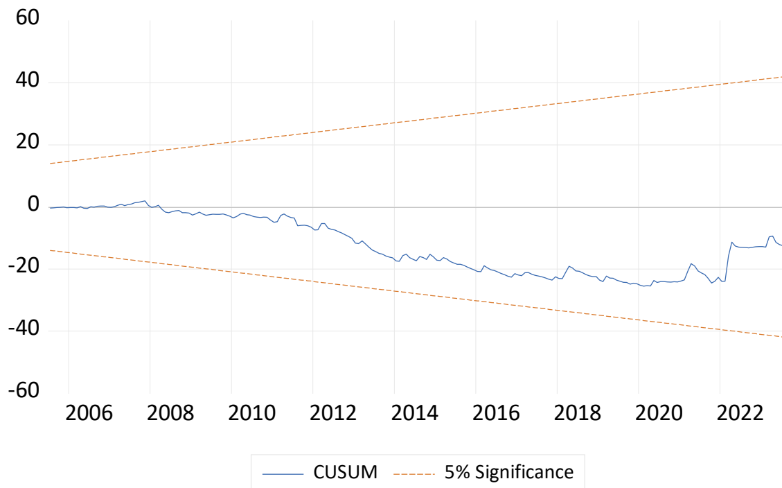
Figura 12. Test de CUSUM
